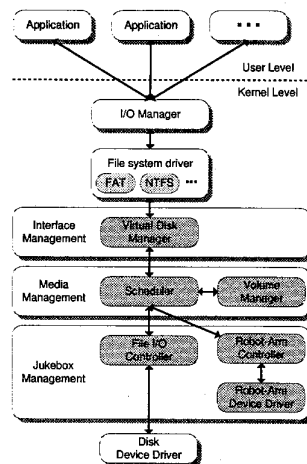
그림 3: 관리 시스템 구성
