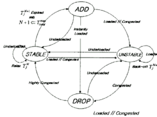
[그림 2] 상태 전이도 (State Transition Diagram)
